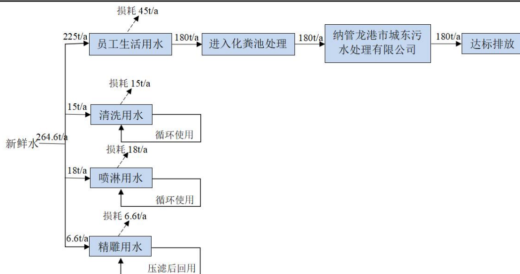
图 2-2 项目水平衡示意图
