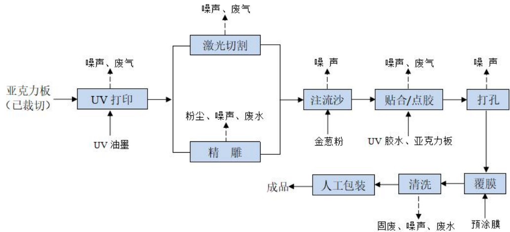
图 2-1 工艺流程图
