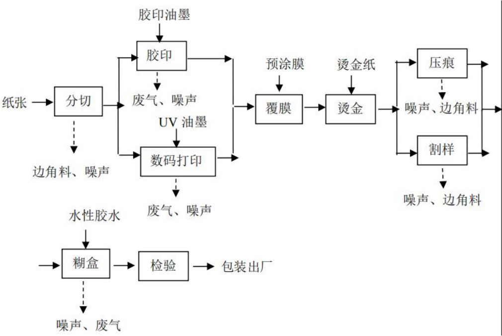
图 2-3 纸盒工艺流程图
