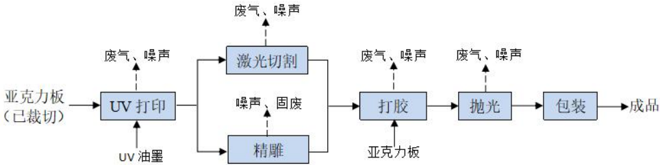
图 2-1 工艺流程图
