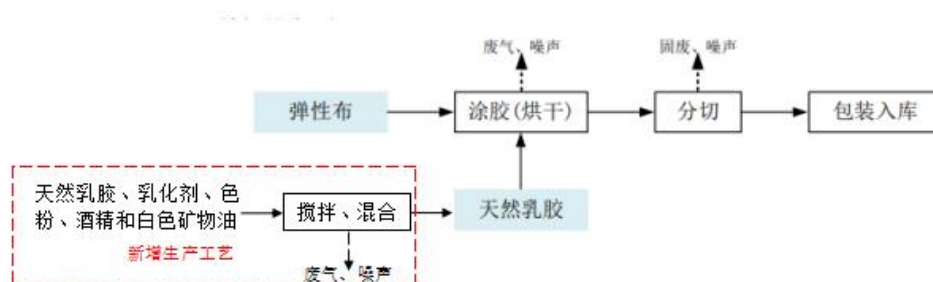
图 2-2 弹性绷带工艺流程图
