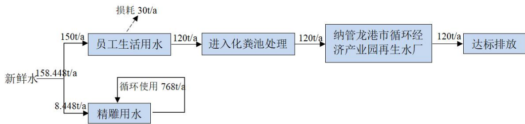
图 2-2 项目水平衡示意图
