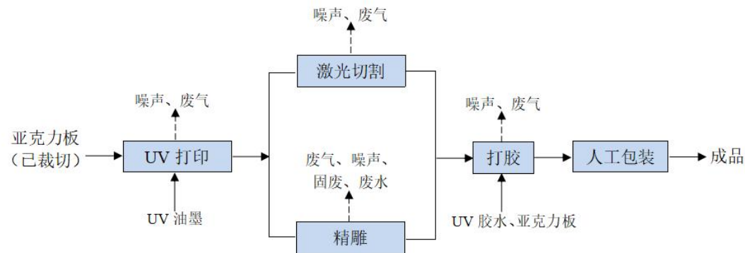
图 2-1 工艺流程图
