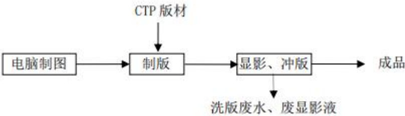
图 2-2 CTP 制版工艺流程图
