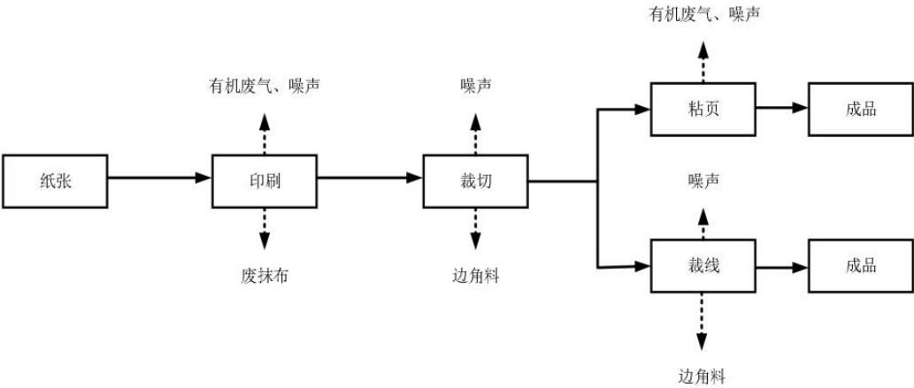
图 2-1 纸制品印刷工艺流程图
