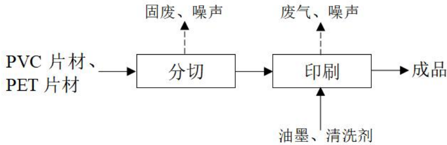
图 2-1 纸制品印刷工艺流程图
