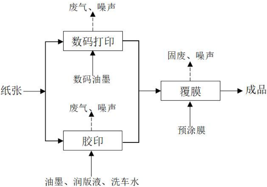
图 2-1 纸制品印刷工艺流程图
