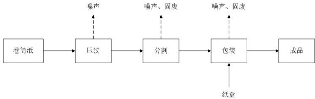
图 2-2 纸盒工艺流程图
