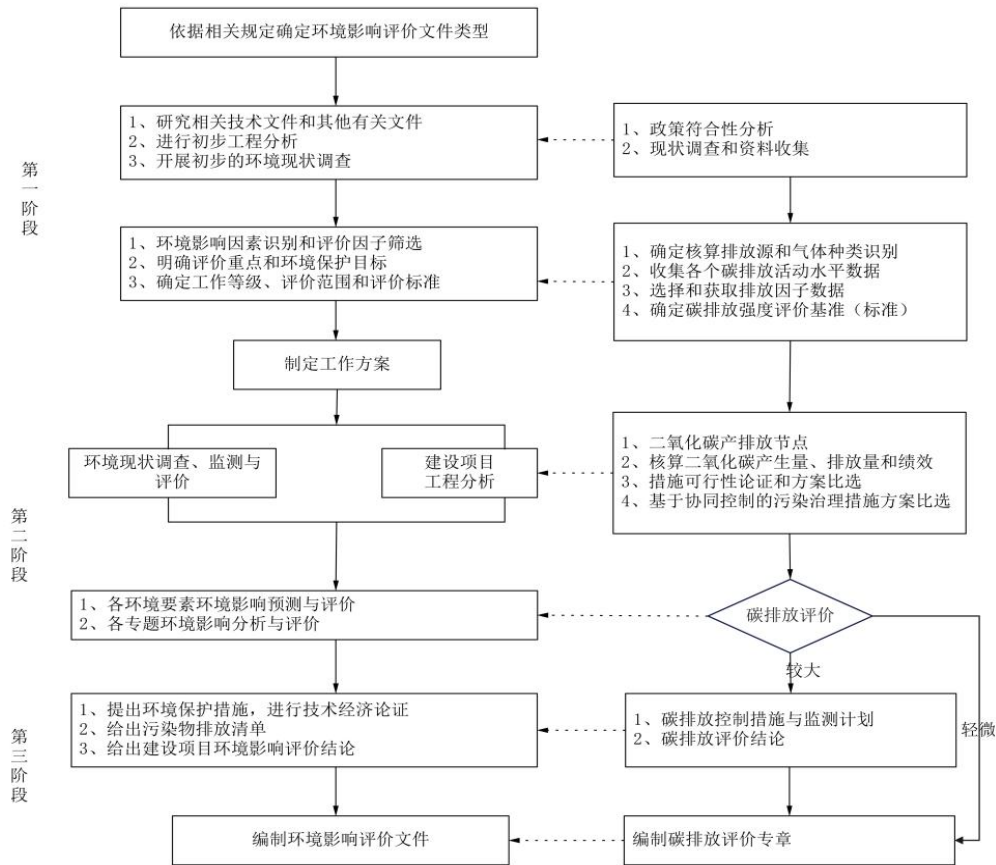
图 4-3 碳排放评价流程
