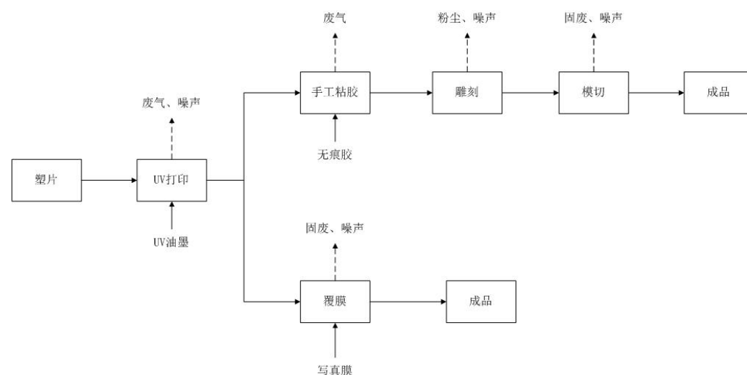
图 2-4 塑料制品生产工艺流程及产污节点图
