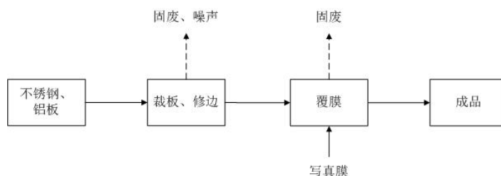
图 2-5 标牌生产工艺流程及产污节点图
