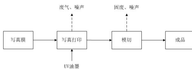
图 2-3 写真膜生产工艺流程及产污节点图
