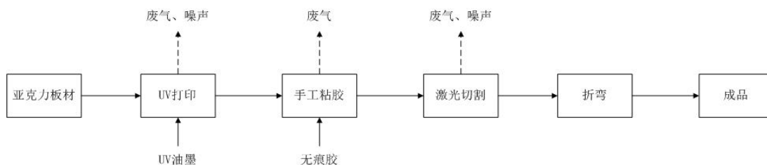
图 2-2 亚克力制品生产工艺流程及产污节点图
