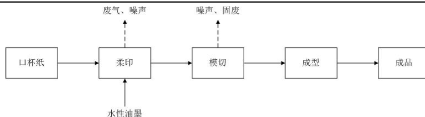
图 2-2 纸杯生产工艺流程图
