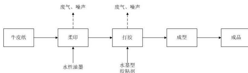
图 2-1 纸袋生产工艺流程图
