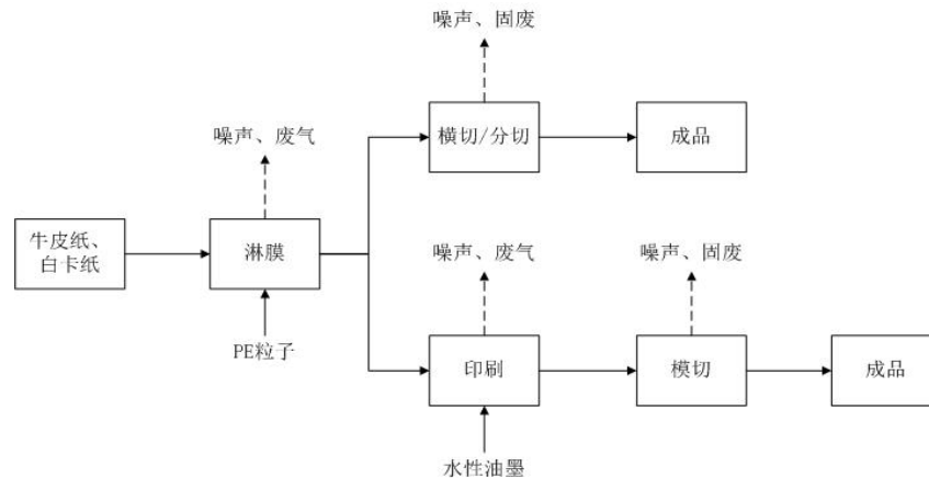
图 2-1 淋膜纸生产工艺流程图
