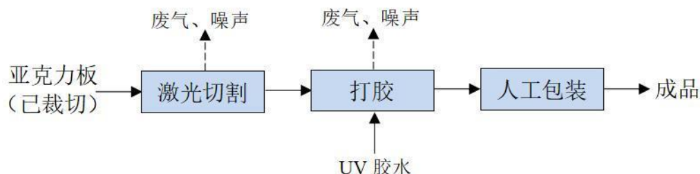
图 3-3 本项目亚克力制品生产工艺流程图
