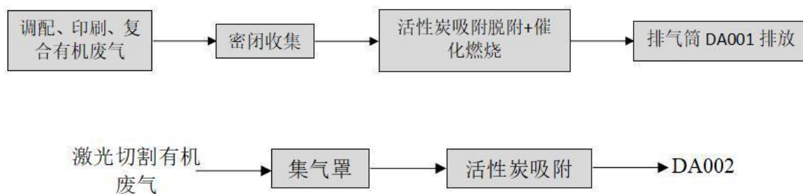
图 6-1 废气处理流程图
