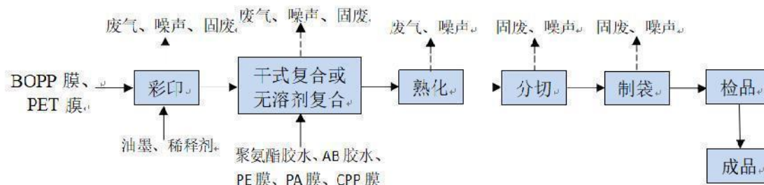
图 3-2 本项目软包装生产工艺流程图
