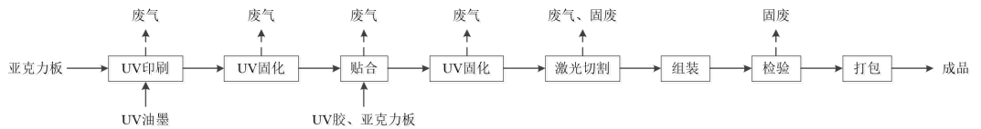
图 2-1 工艺流程图
