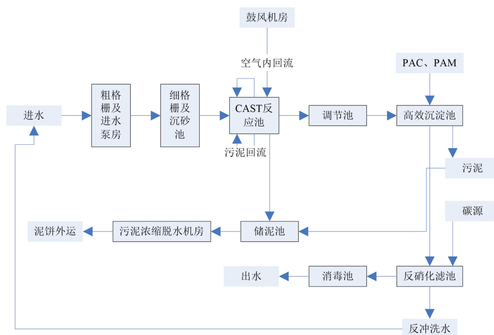
图 4-1 龙港市城东污水处理有限公司工艺流程框图
