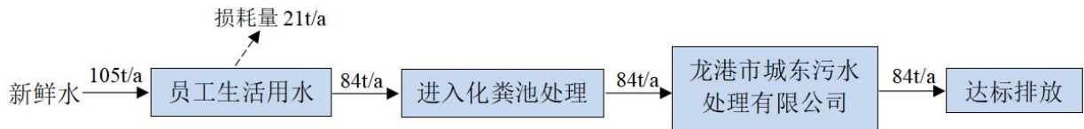
图 3-5 本项目水平衡图
