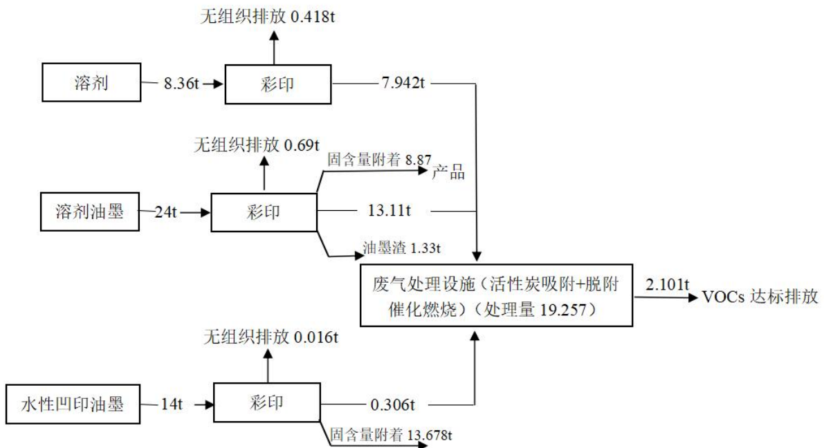
图 3-6 本项目 VOCs 平衡图
