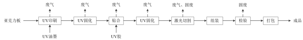
图 2-1 工艺流程图
