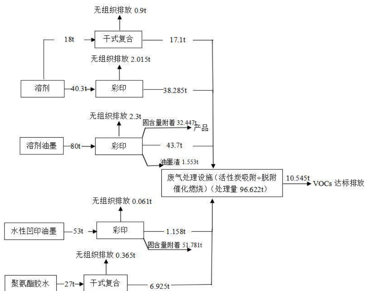
图 3-4 本项目 VOCs 平衡图
