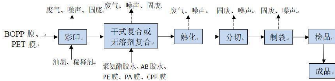
图 3-2 本项目生产工艺流程图
