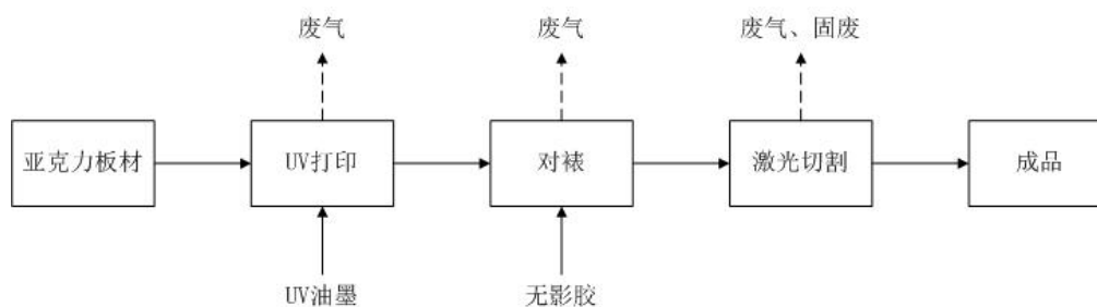
图 2-1 亚克力工艺品工艺流程及产污节点图
