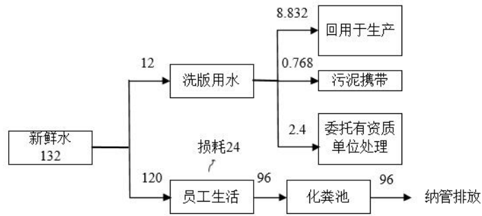
图 2-1 项目水平衡图 (t/a)
