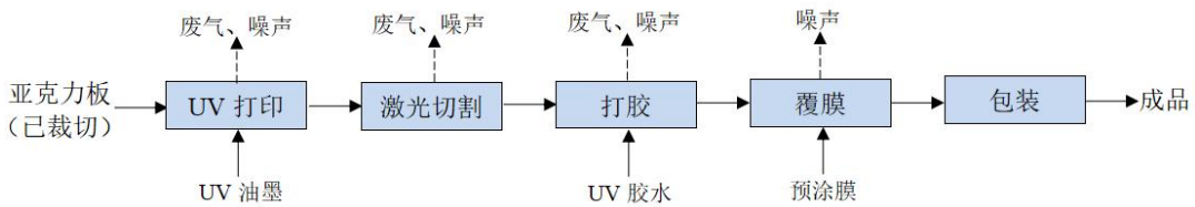
图 2-1 工艺流程图
