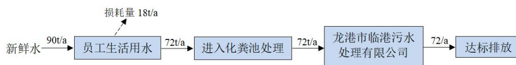
图 2-2 项目水平衡示意图
