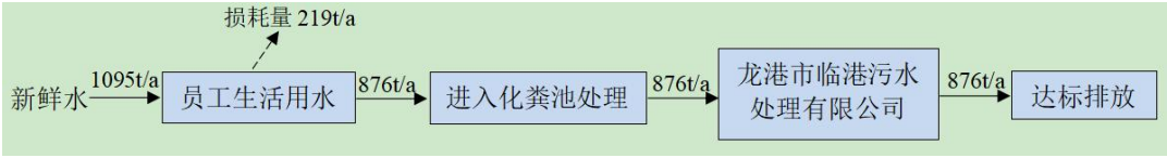
图 2-4 项目水平衡示意图
