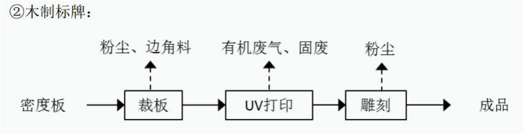
图 2-6 木制标牌工艺流程图
