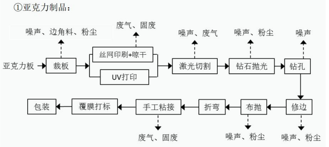
图 2-5 亚克力制品工艺流程图
