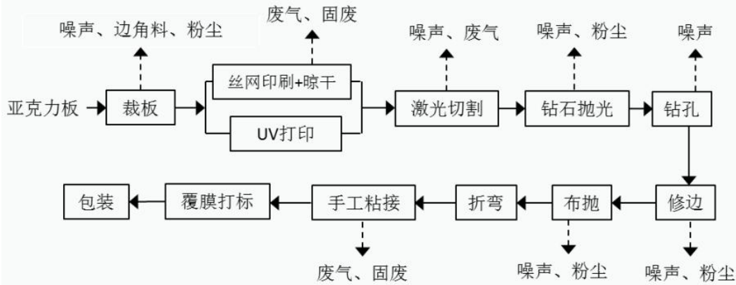
图 2-1 亚克力制品工艺流程图
