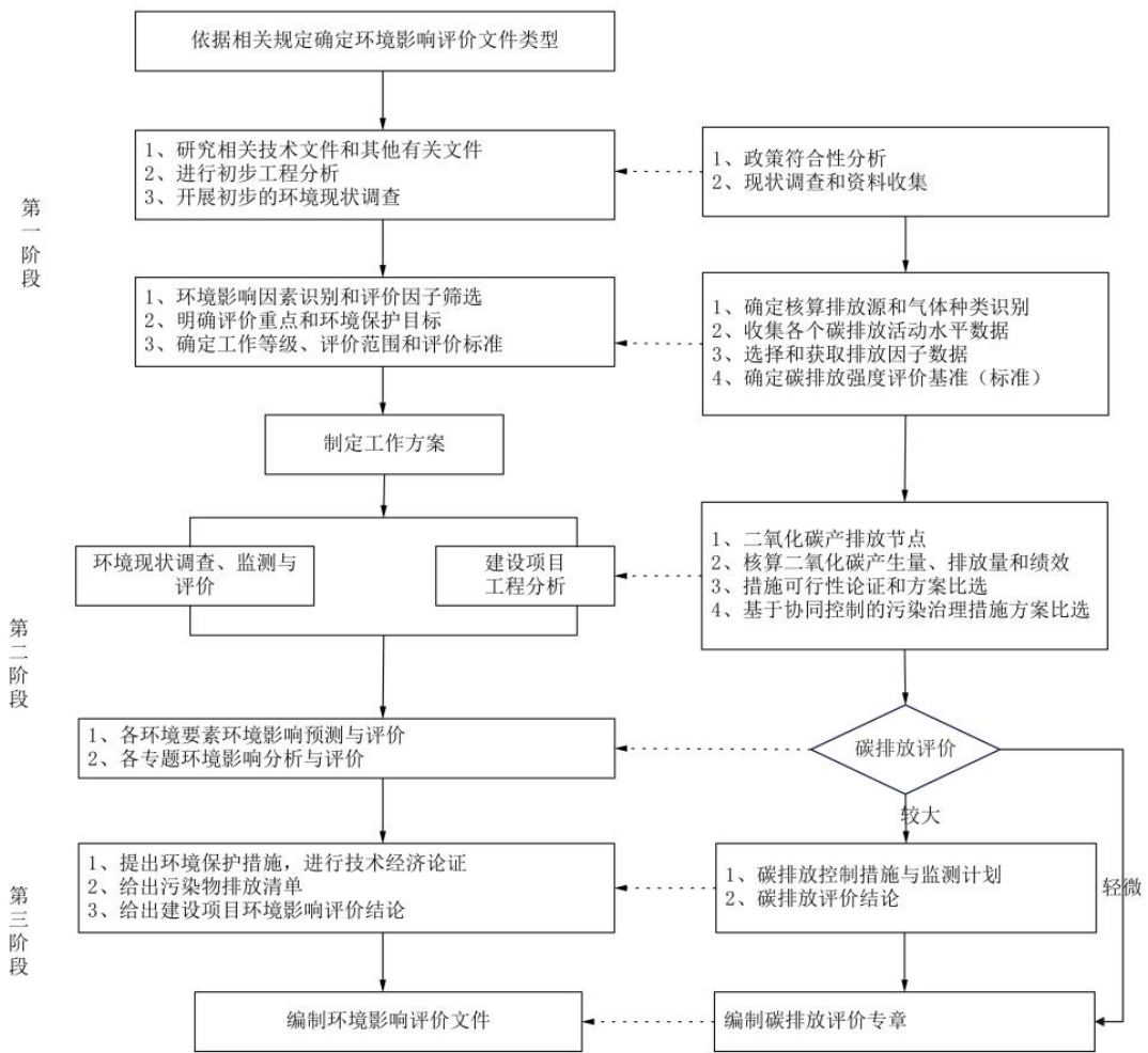
图 4-1 碳排放评价流程
