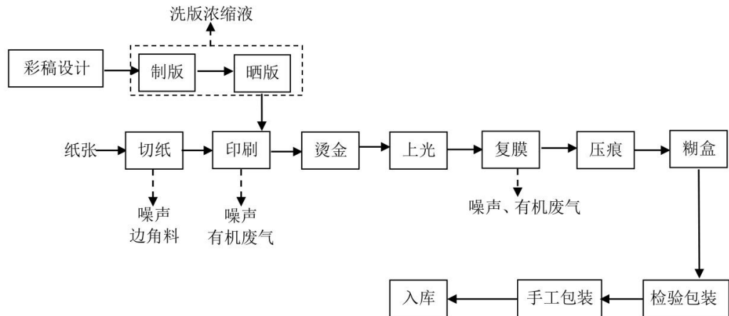
图 2-3 原有项目主要工艺流程产污环节
