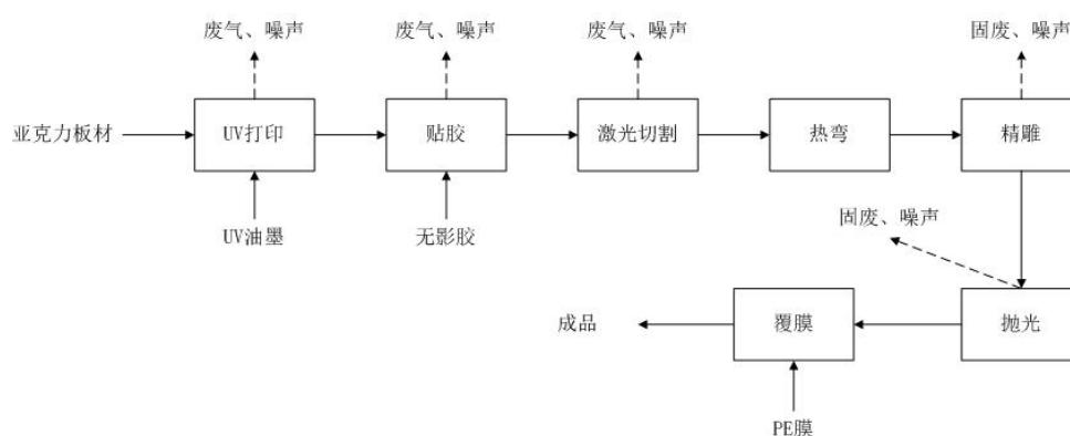
图 2-1 亚克力工艺品工艺流程图
