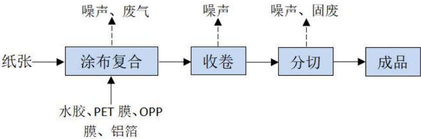
图 2-1 工艺流程图
