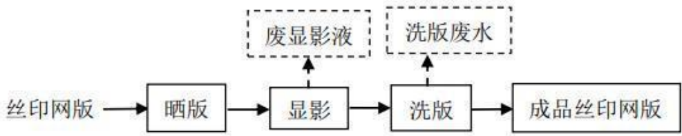
图 2-2 本项目制版流程图
