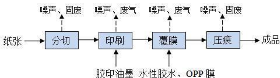
图 2-1 纸制品印刷工艺流程图
