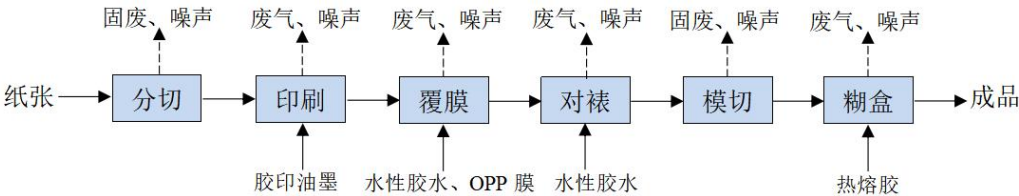
图 2-2 纸盒工艺流程图
