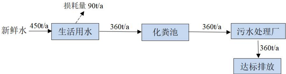
图 2-2 项目水平衡示意图
