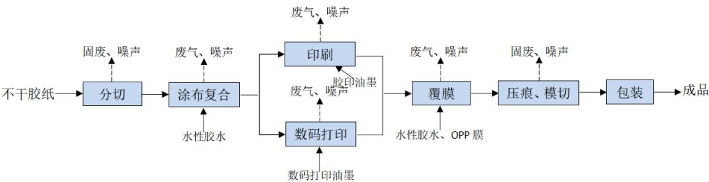
图 2-1 不干胶纸工艺流程图
